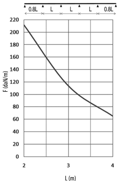
HDKS 60
